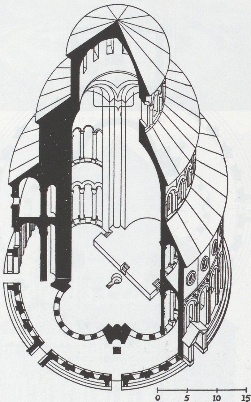
Fig. 14. Zvartnotz, axonométrie d'après Toramanjan.
