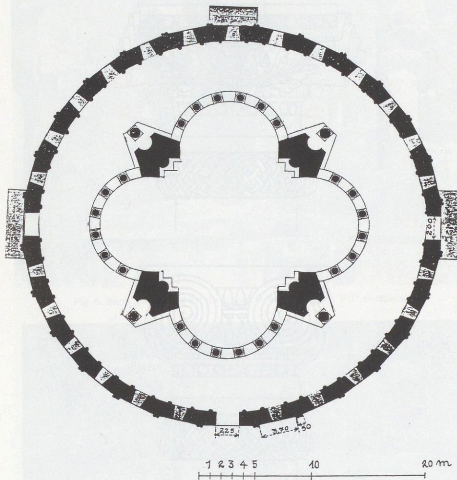
Fig. 3. Bana, plan du tétraconque du VII e siècle, essai de restauration.
