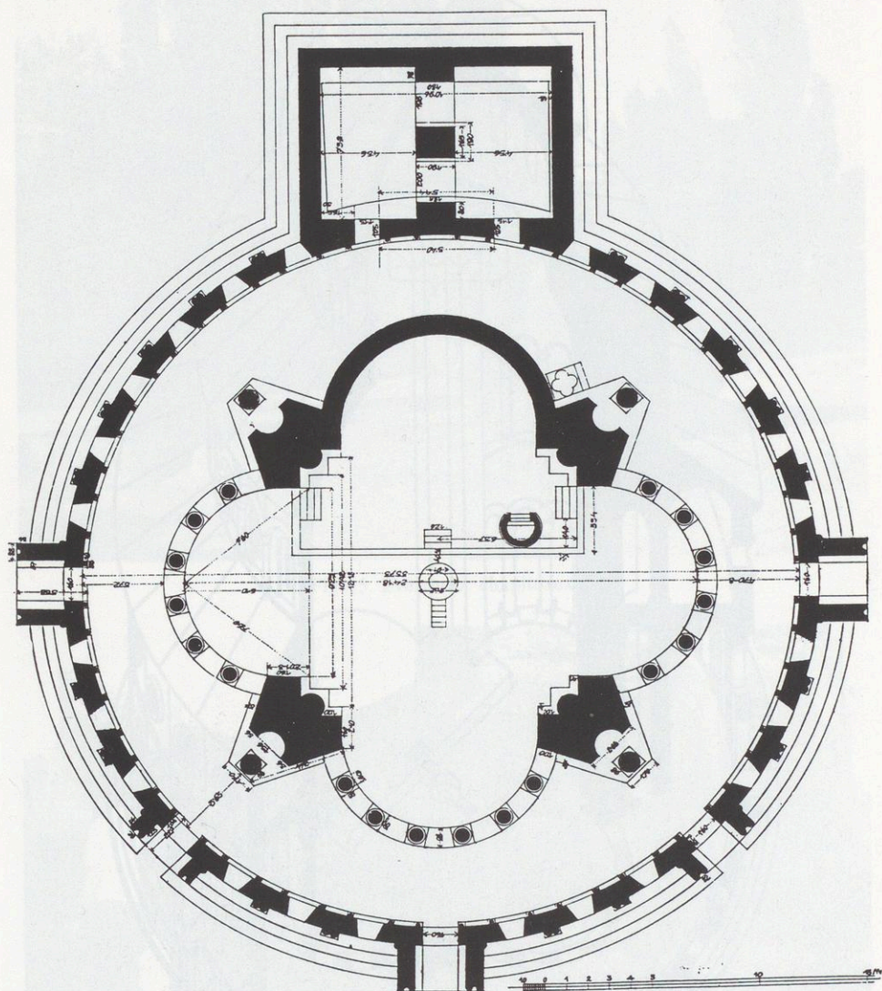
Fig. 12. Zvartnotz, plan d'après Toramanjan.
