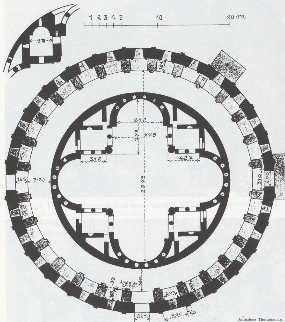
Fig. 2. Bana, plan du tétraconque du X e siècle, d'après Kalgin en 1905: a) étage, b) rez-de-chaussée, pilier nord-est.
